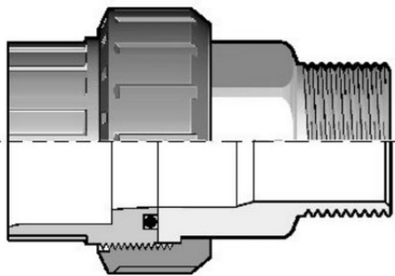
Муфта разборная переходная ХПВХ/ нержавеющая сталь НР 50х1 1/2" PN16
