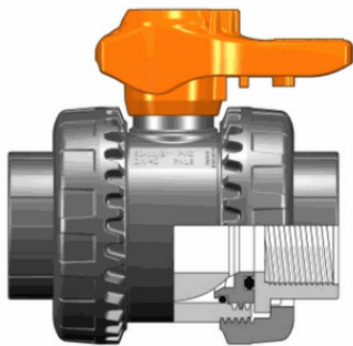
Шаровой кран общего применения VXE ХПВХ с резьбовыми окончаниями R2" (DN50)
