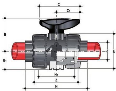
Шаровой кран промышленного применения VKD с муфтовыми окончаниями (уплотнение FKM) PP-H d40 (DN32)
