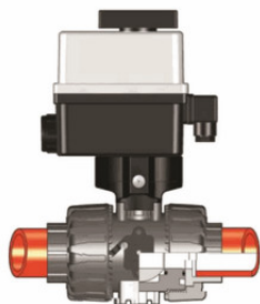
Шаровой кран для регулирования потока VKR с эл.приводом 90-240V, муфтовые окончания (уплотнение EPDM) PP-H d20 (DN15)
