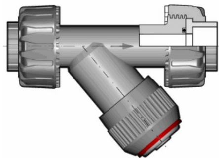
Грязевый фильтр RVUIV PBX с муфтовыми окончаниями, EPDM, FIP d63 (DN50)
