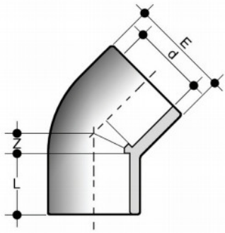
Отвод клеевой 45° ПВХ FIP d200
