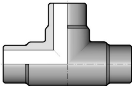
Тройник равнопроходной для стыковой сварки PP-H FIP (PN10) d250 SDR11 PN10
