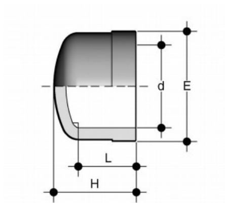
Заглушка клеевая ПВХ FIP d50
