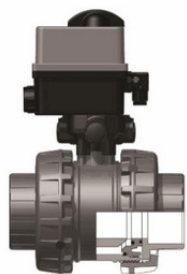
Шаровой кран общего применения VXE ХПВХ с эл.приводом 90-240V, муфтовые окончания d110 (DN90)
