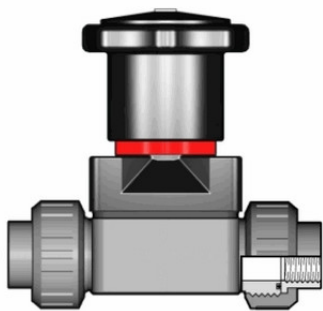
Компактный мембранный клапан CMUFV PBX с разборными муфтовыми окончаниями, EPDM, FIP d15 (DN15)
