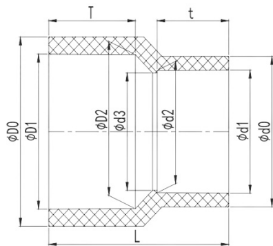
Муфта редукционная ПВХ IPS 400x355
