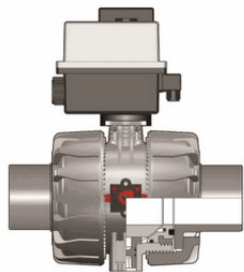
Шаровой кран VKD с эл.приводом 90-240V, втулочные окончания, DN65-100 (уплотнение FKM) PP-H d75 (DN65)
