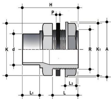
Соединитель с цистерной, LIV ПВХ FIP 32x1 1/4
