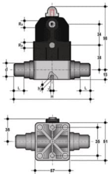
Компактный мембранный клапан CM ХПВХ с пневмоприводом НЗ с втулочными окончаниями d20 (DN15)
