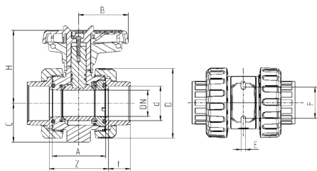
Шаровой кран ПВХ промышленного применения с муфтовыми окончаниями, EPDM, Praher Plastics d75 (DN65)
