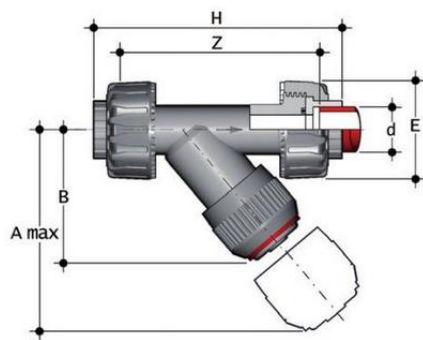
Грязевой фильтр RVUIM с муфтовыми окончаниями (уплотнение EPDM) PP-H d20 (DN15)
