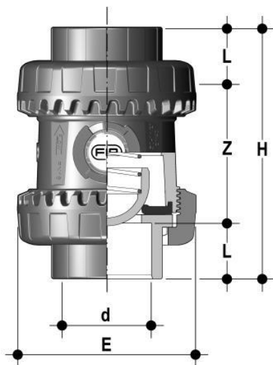
Пружинный шаровой обратный клапан SSEIV ПБХ; с муфтовыми окончаниями, EPDM, FIP d63 (DN50)
