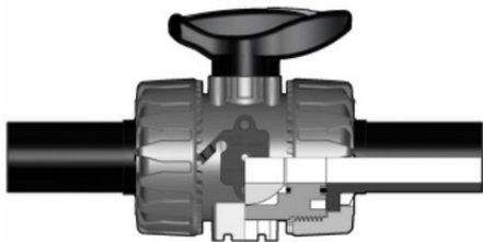
Шаровой кран промышленного применения VKD с патрубками из ПЭ (CVDE) (уплотнение FKM) PP-H d50
