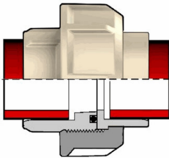
Муфта разборная ПВДФ d20 SDR21 PN16
