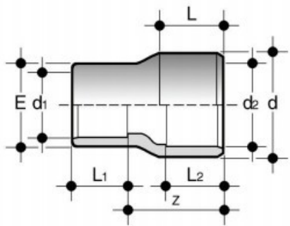
Втулка редукционная ПВХ FIP (трехразмерная) 75х63х63
