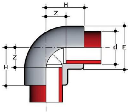
Отвод ПВДФ 90° d40 SDR21 PN16
