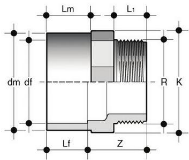
Ниппель переходной с НР ХПВХ 25x20x1/2" PN16
