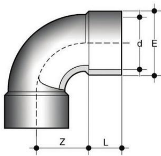
Отвод 90° ХПВХ d225 PN16
