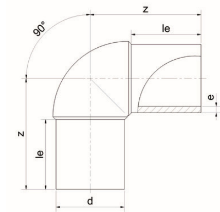
Отвод 90° PP-H Simona d110 SDR11 PN10
