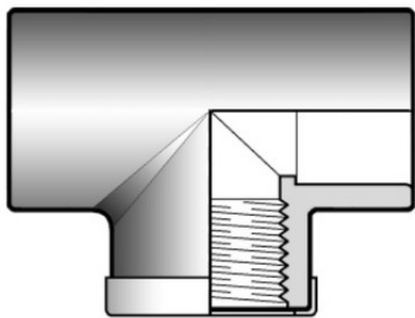
Тройник переходной с НР ПВХ FIP 63x2
