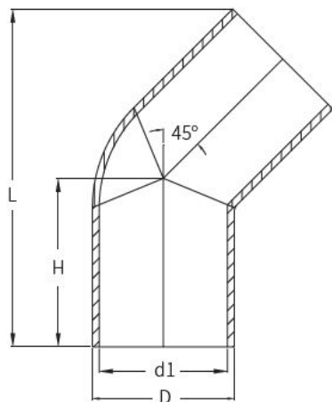
Отвод для стыковой сварки ПВДФ 45° d25 PN 16
