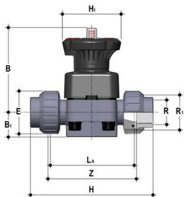
Мембранный клапан ДК ХПВХ с разборными резьбовыми окончаниями R2" (DN50)
