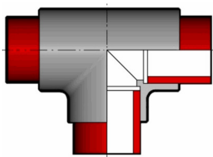
Тройник ПВДФ 90° d63 SDR21 PN16
