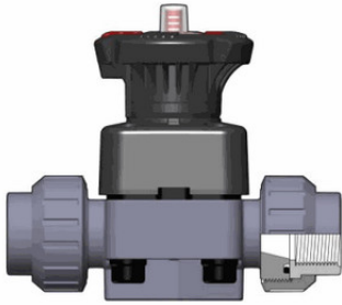
Мембранный клапан DKUFV ПВХ с резьбовыми окончаниями, FKM, FIP R1/2" (DN15)
