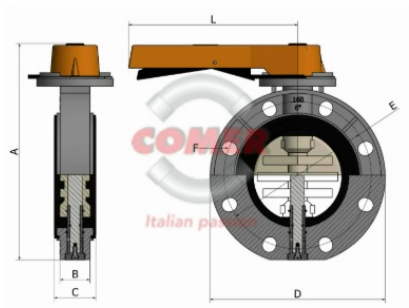
Дисковый затвор ПВХ с рукояткой, EPDM, Comer d140 (DN125)
