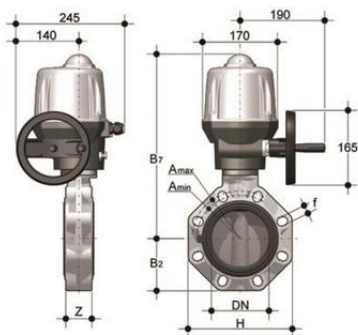
Дисковый затвор FK ПВДФ с эл.приводом 24V AC/DC d140 (DN125)
