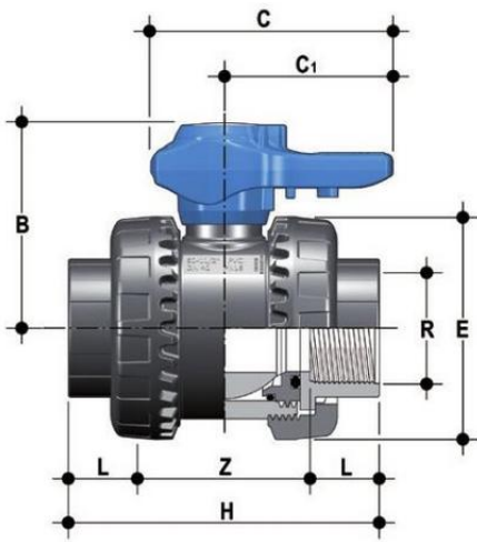
Шаровой кран ПВХ общего применения VEE; муфтовые окончания с ВР, EPDM, FIP R4" (DN100)
