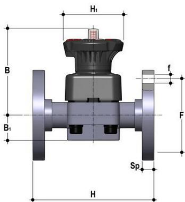
Мембранный клапан DKOM с фланцевыми окончаниями (уплотнение РТFЕ / мембрана РТFЕ) РР-Н d40 (DN32)
