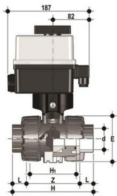
Шаровой кран для регулирования потока VKR ПБХ с эл.приводом 24V AC 12VDC, муфтовые окончания, FKM, FIP d16 (DN10)
