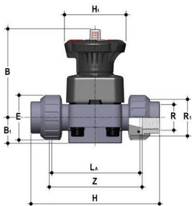
Мембранный клапан DKUFV ПВХ с резьбовыми окончаниями, PTFE, FIP R1/2" (DN15)
