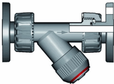
Грязевой фильтр RV ХПВХ с фланцевыми окончаниями d40 (DN32)
