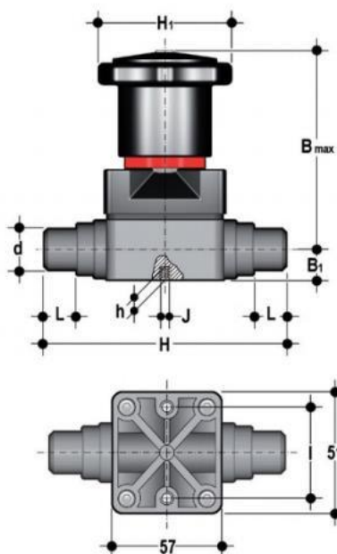
Компактный мембранный клапан CMDV PBX с втулочными окончаниями, EPDM, FIP d20 (DN15)
