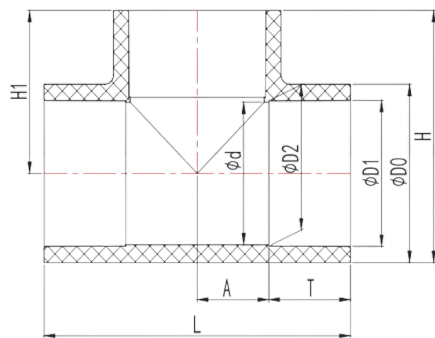
Тройник равнопроходной клеевой 90° ПВХ IPS d32
