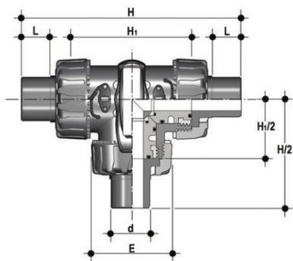
3-х ходовой шаровой кран ПВХ ТКД с втулочными окончаниями, L-шар, EPDM, FIP d32 (DN25)
