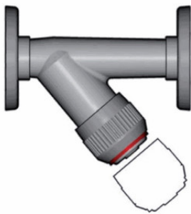
Грязевой фильтр RVOM с фланцевыми окончаниями (уплотнение FKM) PP-H d75 (DN65)
