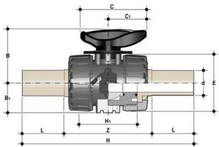
Шаровой кран для регулирования потока VKR с патрубками (CVDM) (уплотнение EPDM) PP-H d50 (DN40)
