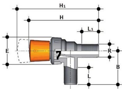
Мембранный кран RMRV ПВХ, резьбовое соединение, EPDM, FIP d15 (DN15)
