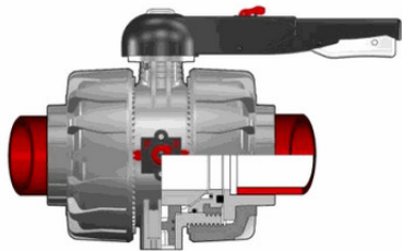
Шаровой кран промышленного применения VKD С муфтовыми окончаниями (уплотнение FKM) PP-H d90 (DN80)
