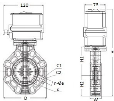
Дисковый затвор IFK PP-H с электрическим приводом 24V DC, FKM, IPS d90 (DN80)
