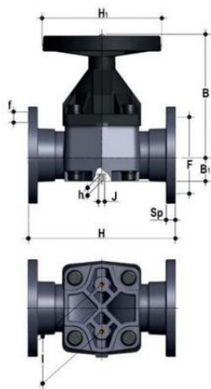
Мембранный клапан VMOV PBX с фланцевыми окончаниями, PTFE, FIP d90 (DN80)
