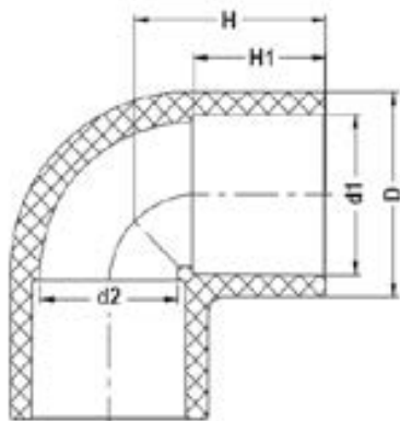
Отвод ПВДФ 90° (IPS) d75 PN 16
