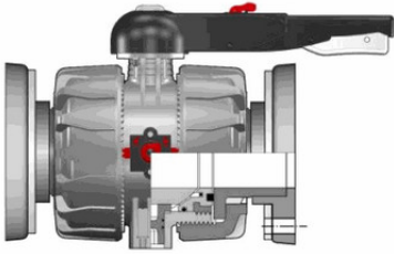
Шаровой кран промышленного применения VKD С фланцевыми окончаниями (уплотнение EPDM) PP-H d110
