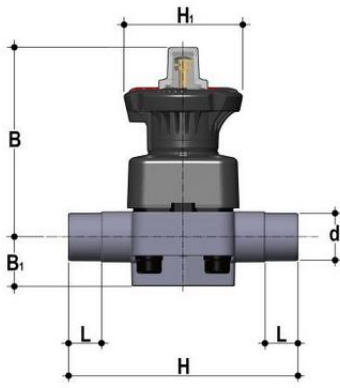
Мембранный клапан DK/L ХПВХ с втулочными окончаниями d25 (DN20)
