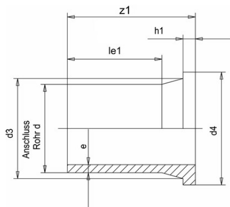
Бурт PP-H Simona d90 SDR11 PN10
