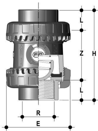
Пружинный шаровой обратный клапан SSEFV ПБХ; с резьбовыми окончаниями, EPDM, FIP R3/4" (DN20)
